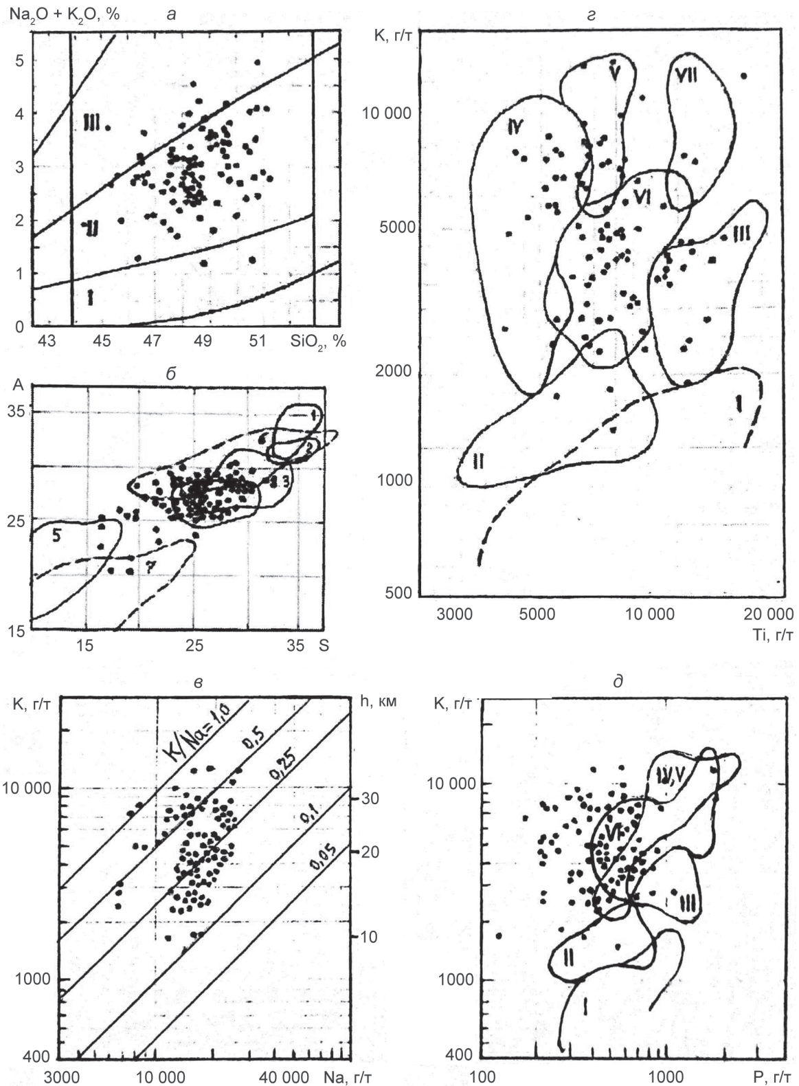
Рис. 6. Положение химических составов метабазальтов Сутамского блока раннего архея Алданского щита на классификационных (а – \text{SiO}_2 - (\text{K}_2\text{O} + \text{Na}_2\text{O}) ; б – \text{A-S} ; в – \text{K-Na} ) и геодинамических (г – \text{K-Ti} ; д – \text{K-P} ) диаграммах
