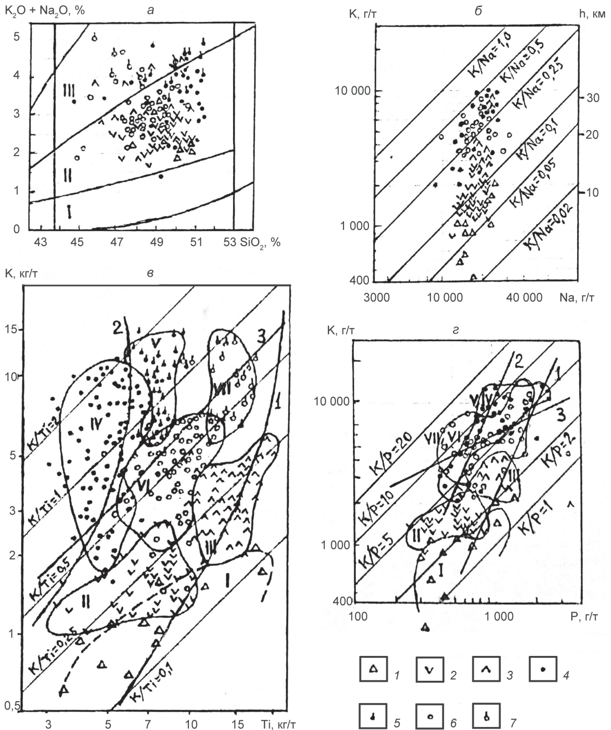
Рис. 2. Положение химических составов базальтов различных современных и мезозой-кайнозойских геодинамических обстановок на петрохимических (а – классификационной SiO_2 - (K_2O + Na_2O) ; б – K–Na) и геодинамических (в – K–Ti; з – K–P) диаграммах
