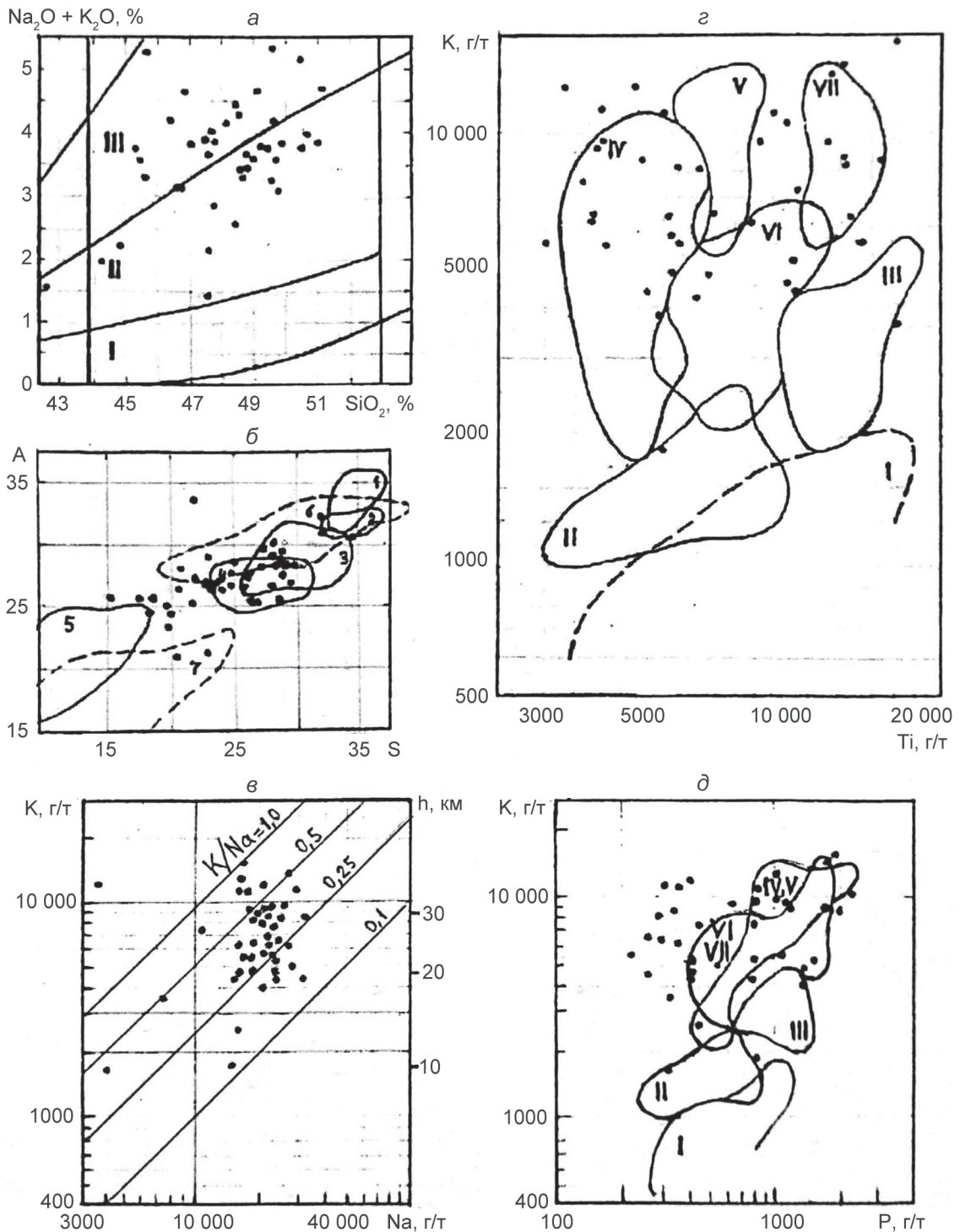
Рис. 7. Положение химических составов метабазальтов Нимырьской структурно-формационной зоны раннего архея Алданского щита на классификационных (а – SiO 2 – (K 2 O + Na 2 O); б – А–S; в – К–Na) и геодинамических (г – К–Ti; д – К–P) диаграммах
