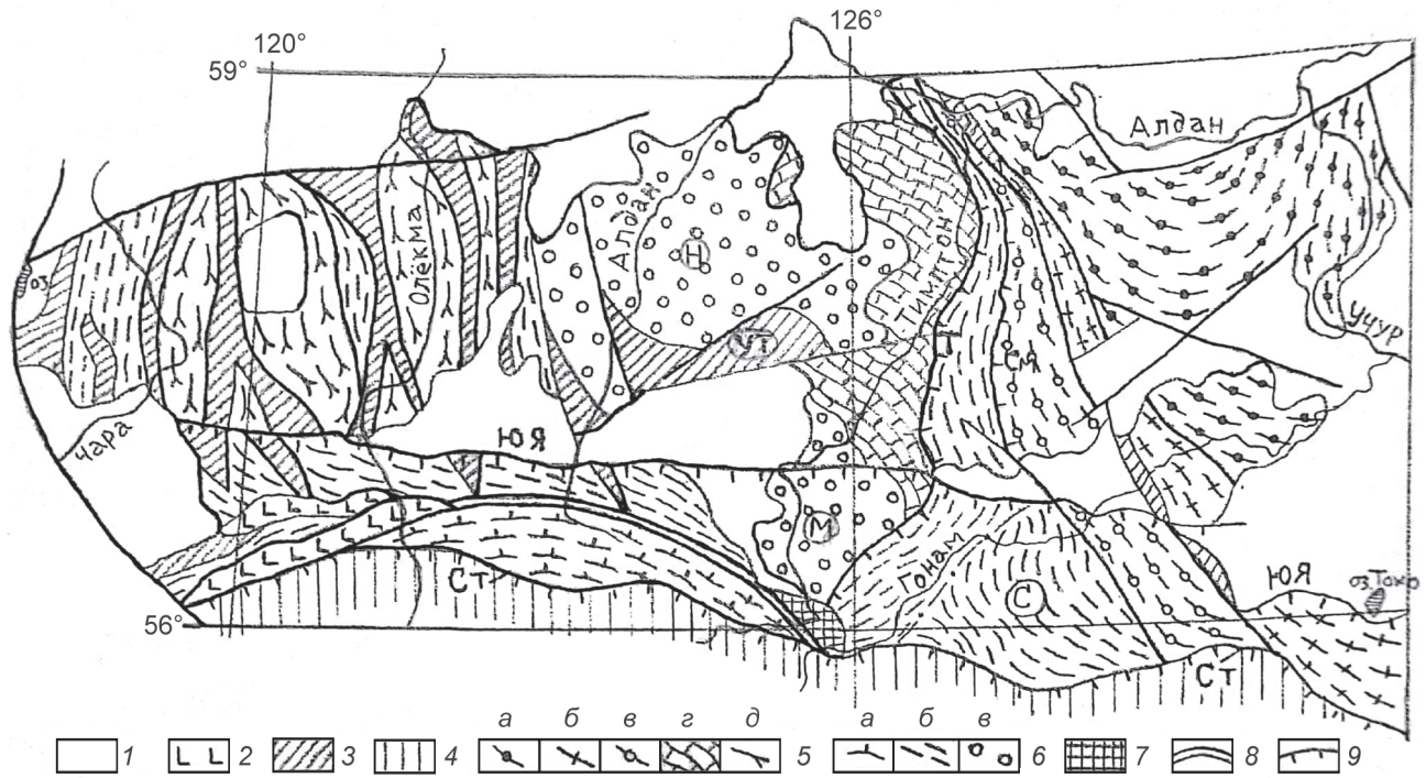
Рис. 1. Тектоническая схема архейд Алданского щита
