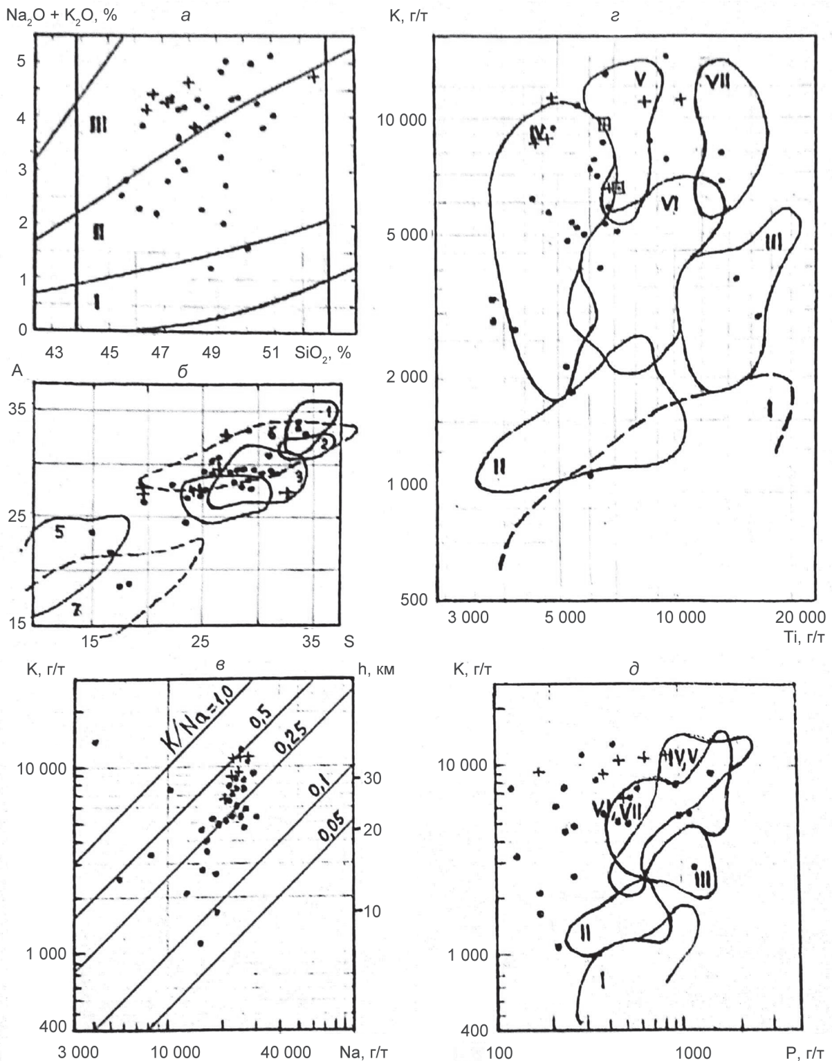
Рис. 3. Положение химических составов метабазальтов Тантракского блока катархей Алданского щита на классификационных (а – \text{SiO}_2 - (\text{K}_2\text{O} + \text{Na}_2\text{O}) ; б – А–S; в – К–Na) и геодинамических (г – К–Ti; д – К–P) диаграммах
