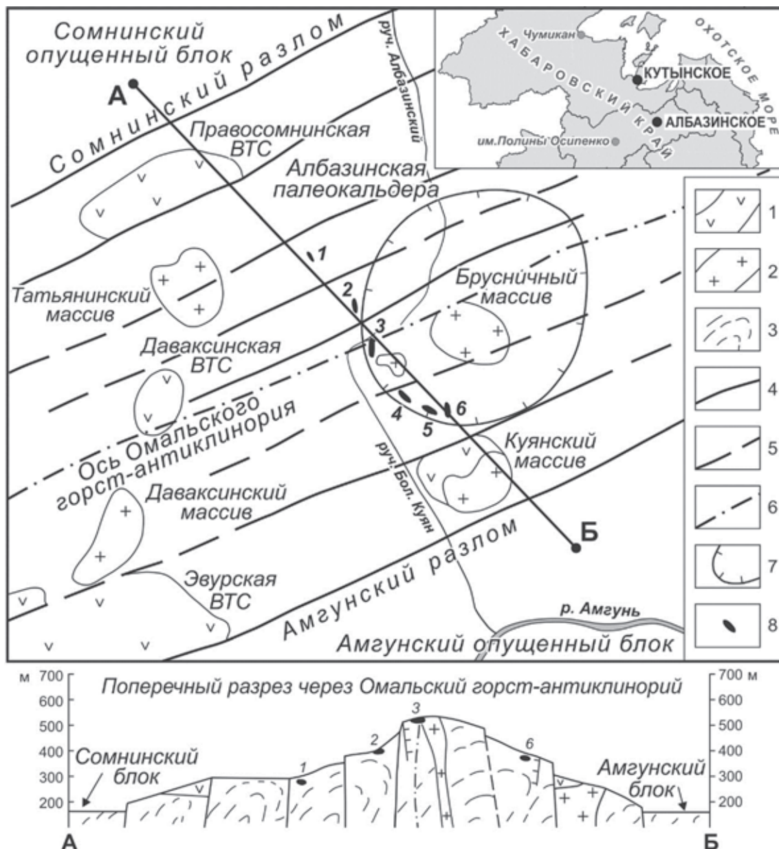
Рис. 1. Схема Омальского горст-антиклинария и его поперечный разрез
