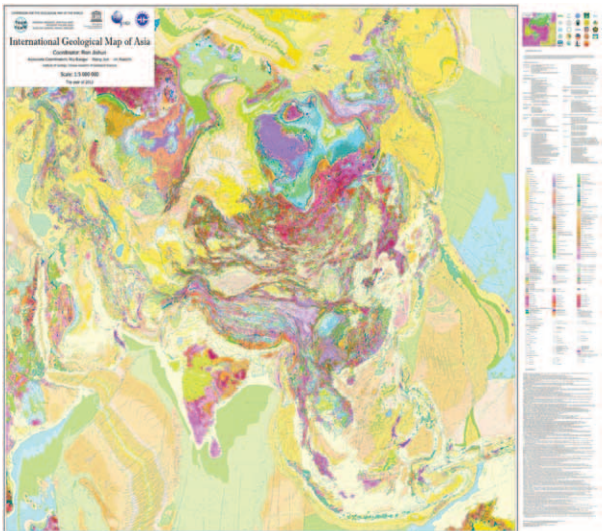
Рис. 11. Международная геологическая карта Азии масштаба 1 : 5 000 000 – IGMA-5000 (Китай, 2012)
