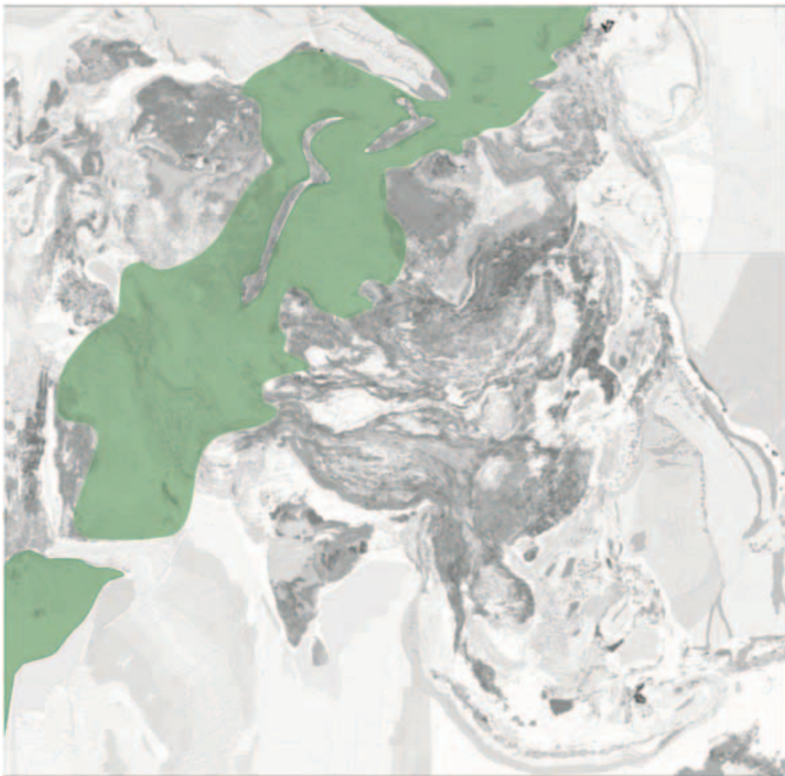
Рис. 12. Положение Палеоазиатского океанического бассейна в структурах Евразии (пояснения в тексте)
