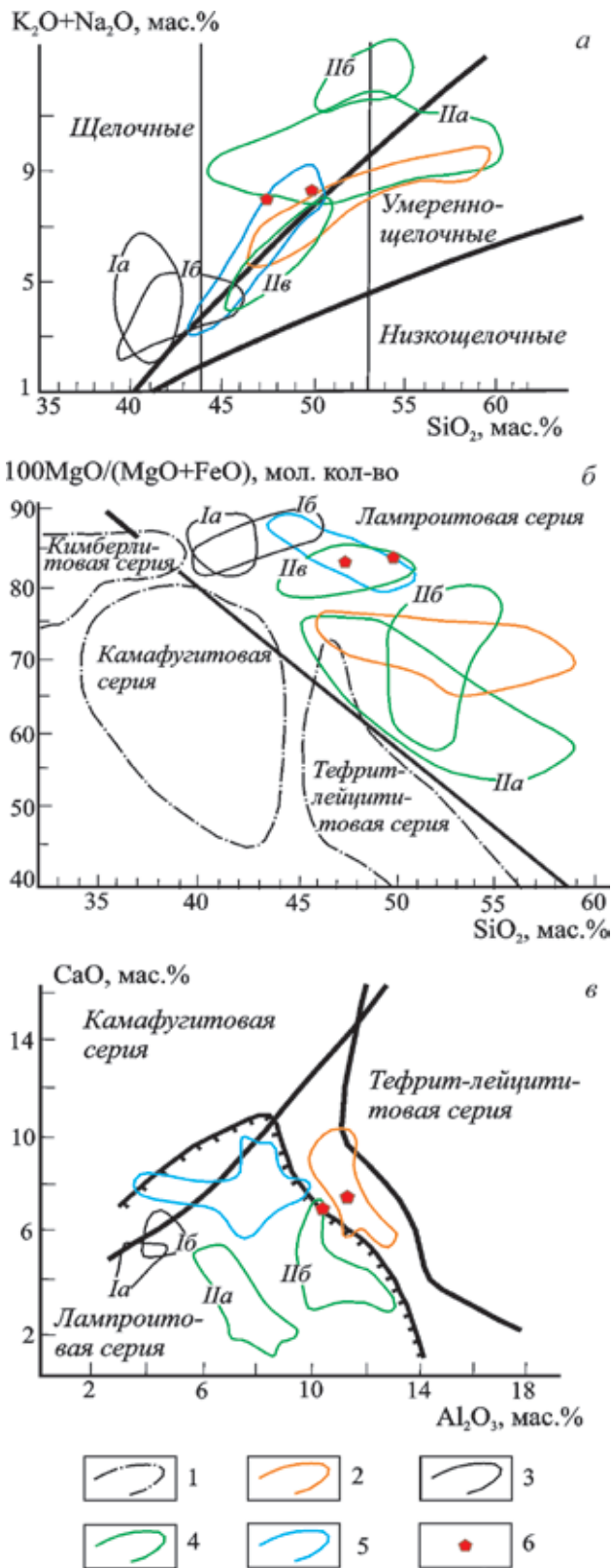
Рис. 6. Классификационные диаграммы соотношений окислов в породах калиевых серий: \text{K}_2\text{O} + \text{Na}_2\text{O} и \text{SiO}_2 – а; \text{SiO}_2 (мас.%) и \text{mg}' (мол. кол-во) – б; \text{CaO} и \text{Al}_2\text{O}_3 – в
