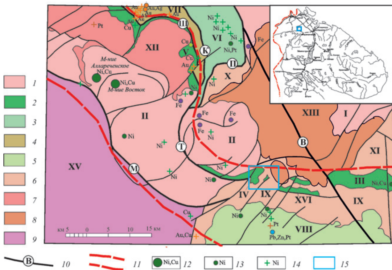
Рис. 1. Тектоническая схема Солонзерской площади (А. Б. Дуракова, А. М. Ремизова, 2002 с авторскими дополнениями)
