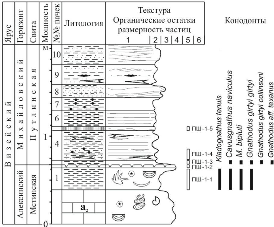
Разрез пограничных отложений мстинской и путлинской свит между дер. Путлино и Шиботово
