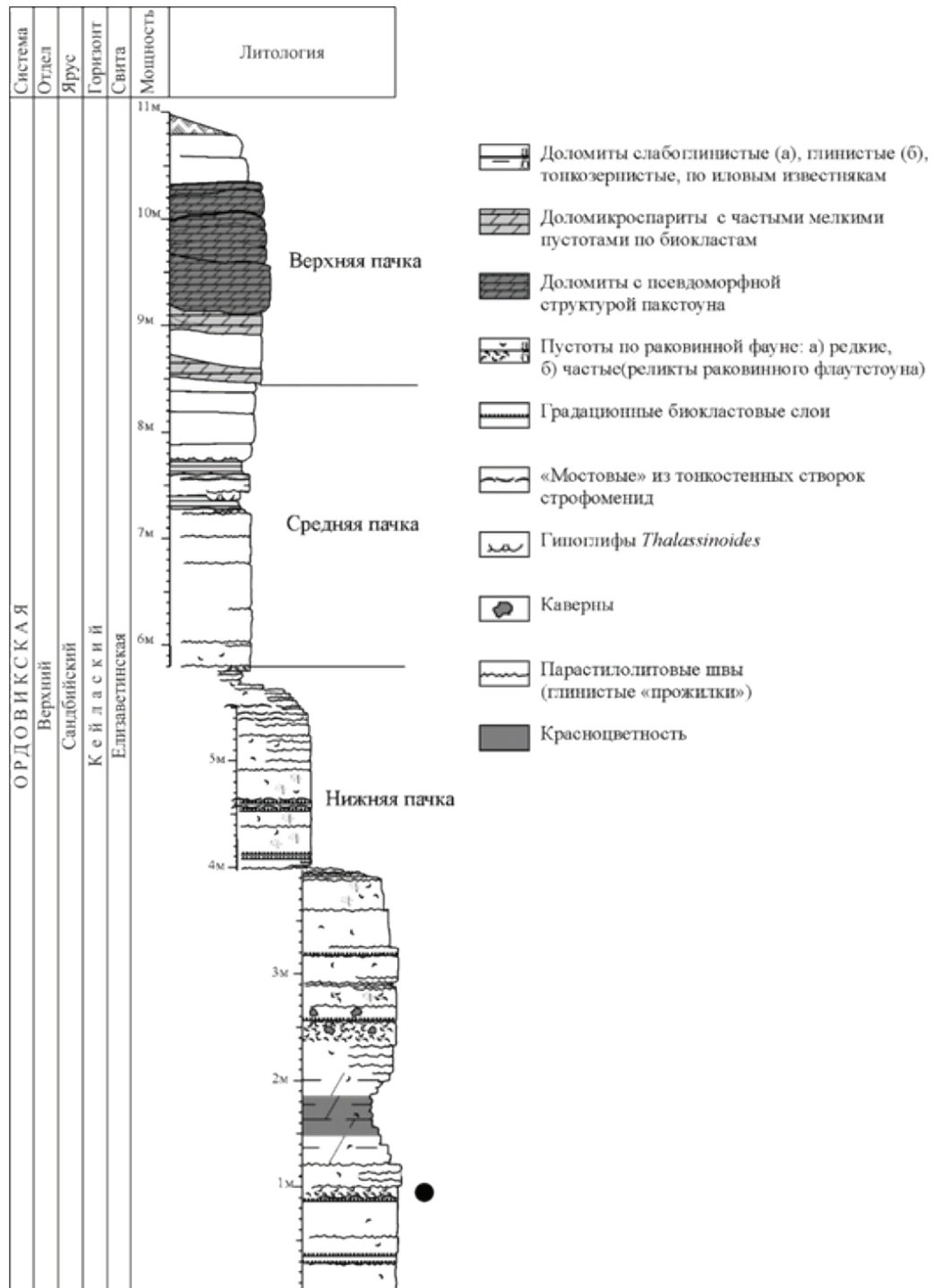
Разрез средней части елизаветинской свиты в карьере Елизаветино. Точкой отмечен уровень пробы К1-1, проба К1-0 расположена на 2 м ниже
