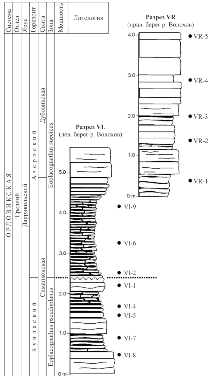
Литологическая колонка нижней части азериского горизонта
