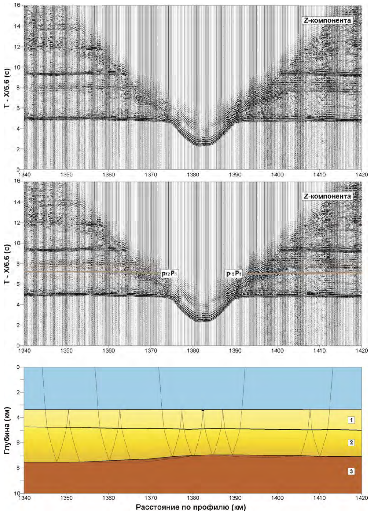
Рис. 15. Лучевое моделирование кратных волн, p_{12}P_3 -волна (ПК 1382, модель_1)
