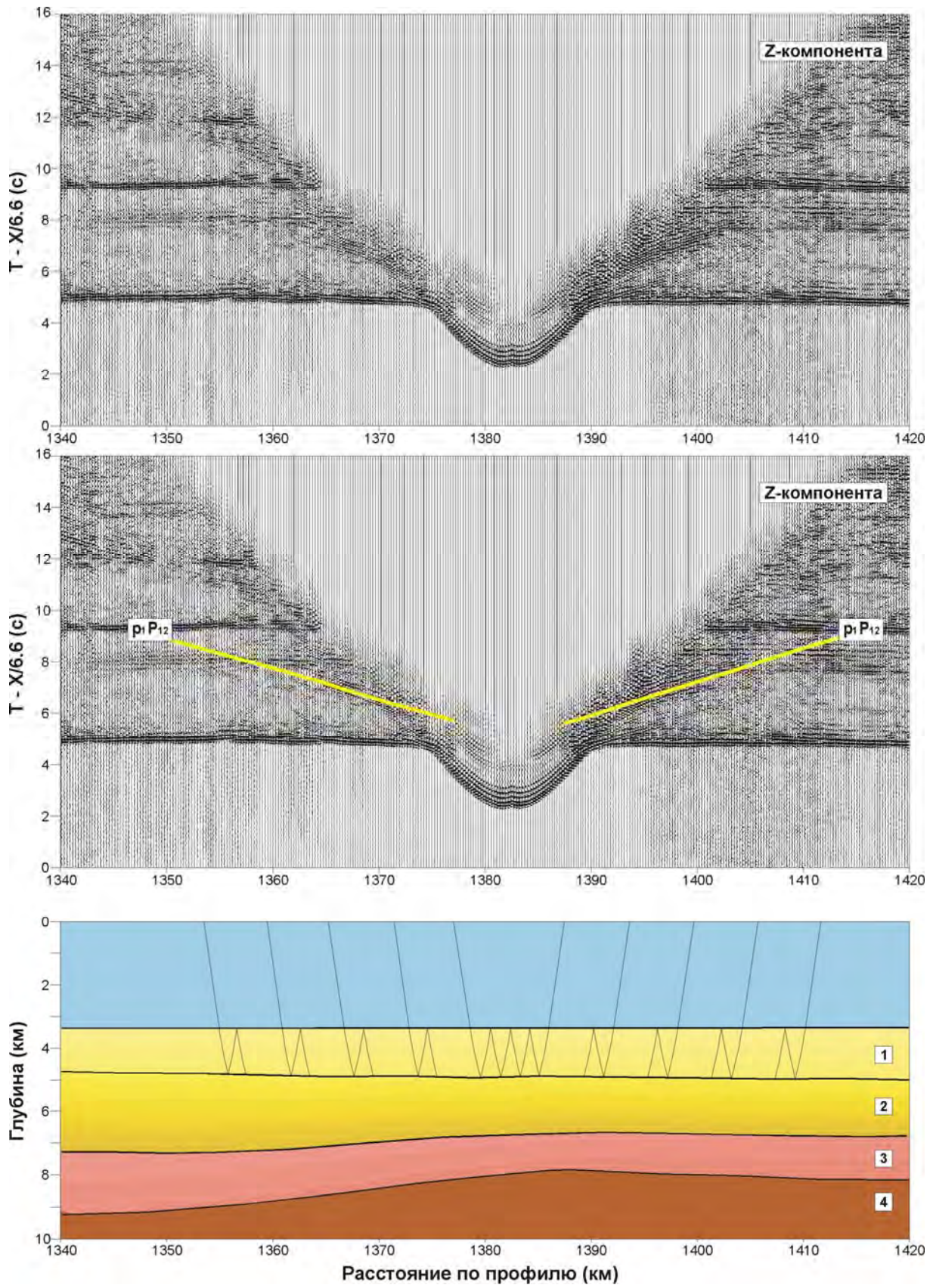
Рис. 14. Лучевое моделирование кратных волн, P_1P_{12} -волна (ПК 1382, модель_2)
