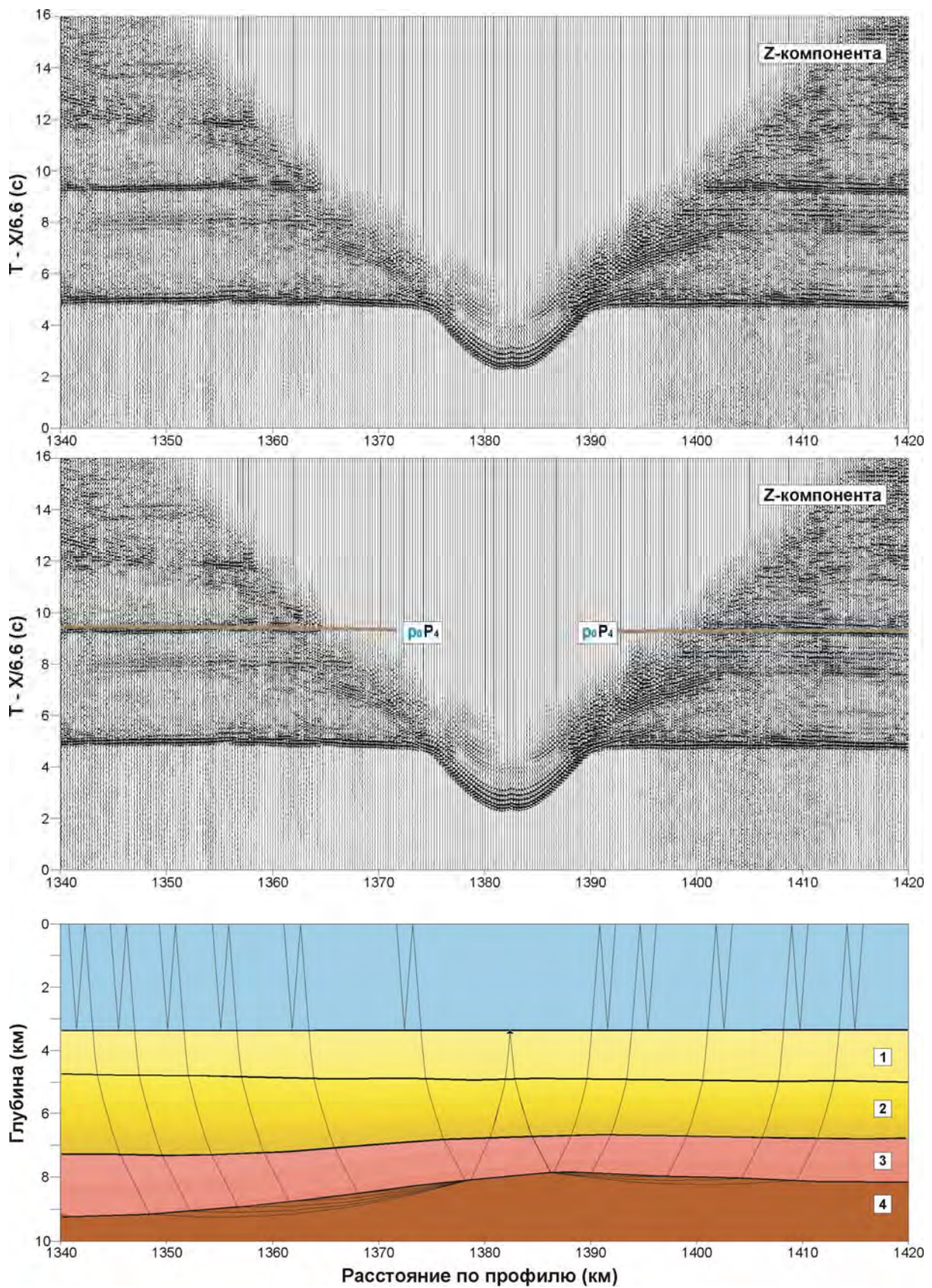
Рис. 8. Лучевое моделирование кратных волн, связанных с водным слоем, p_0P_4 -волна (ПК 1382, модель_2)
