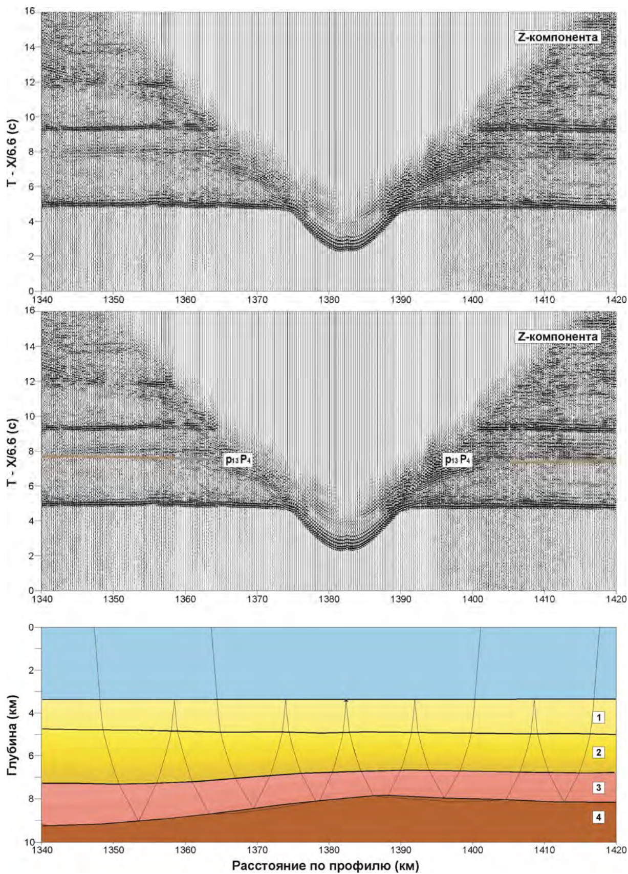
Рис. 16. Лучевое моделирование кратных волн, p_{13}P_4 -волна (ПК 1382, модель_2)
